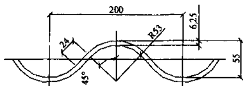
Рис. А.5. Профиль гофрированного листа Толщина листа 4,0-7,10 мм
