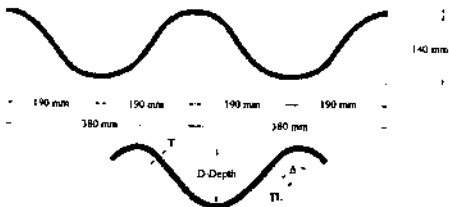
Рис. А.4. Профиль гофрированного листа Толщина листа 3,5-7,1 мм, углы изгиба гофра 49,75-50,43^\circ Прямая оставка 110,78-106,15 мм
