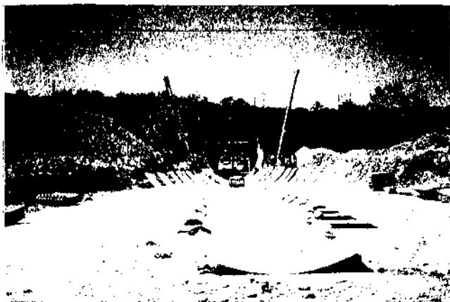
Рис. 20. Сборка МТТ из отдельных элементов
