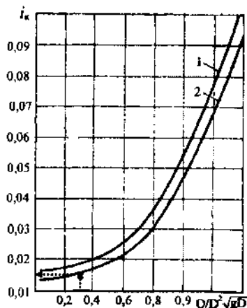
Рис. 5.27. График для определения критического уклона i_k для круглых гофрированных труб с гладкими лотками ( n_{кр} = 0,025 ): 1 – D = 1,5 м; 2 – при D = 2,0 м
