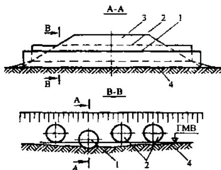
Рис. б. Многоочковое водопропускное сооружение из МГС с расположением очков в разных уровнях:
